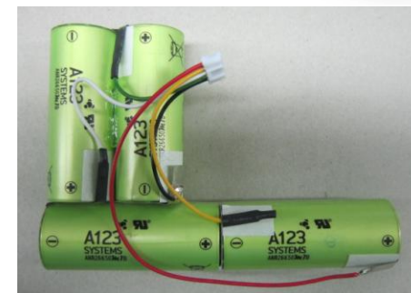
A123 APR26650M1 4S1P
